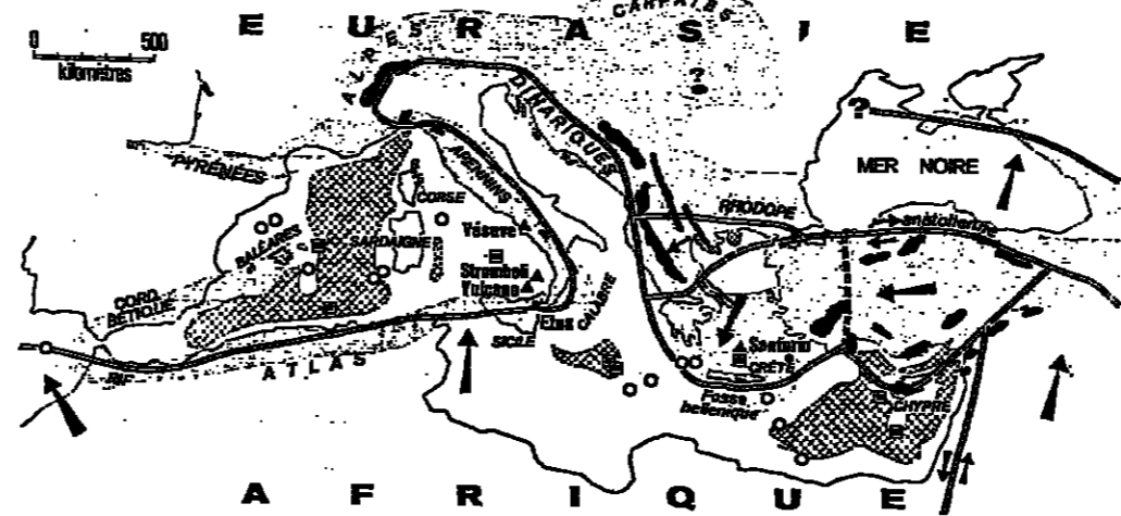
○ Sites des forages de 1970 ■ Sites prévus des forages de 1975 ■ Evaporites épaisses de plus de 1000 mètres ■ Zones fissées — Limites actuelles des plaques — Limites supposées des plaques
